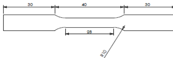
Fig. 3. Configuration ASTM E21
