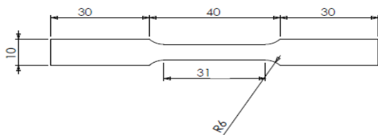
Fig. 2. Configuration ASTM E8
